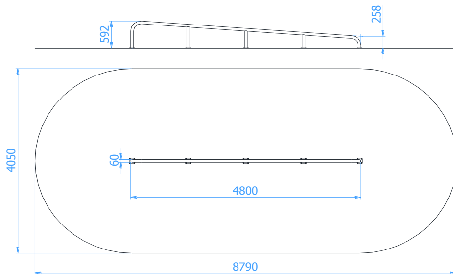
Wymiary urządzenia
