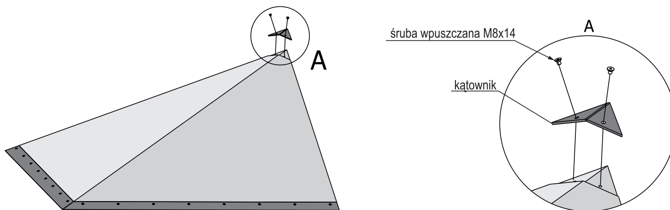
Rys. 2 Sposób mocowania kątownika ochronnego.
