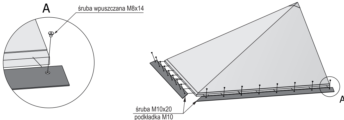
Rys. 1 Sposób mocowania szpiców.
