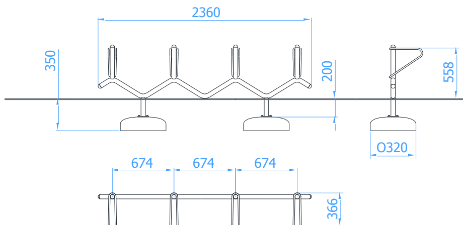
Wymiary urządzenia
