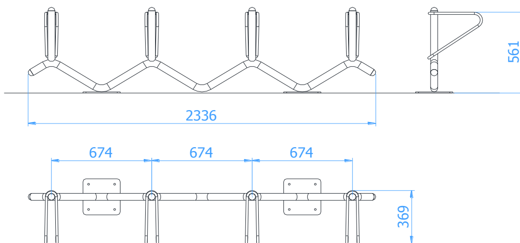
Wymiary urządzenia
