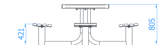
Wymiary urządzenia
