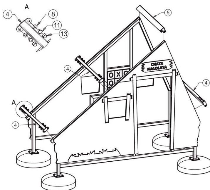
Rys. 2 Schemat łączenie boków.
