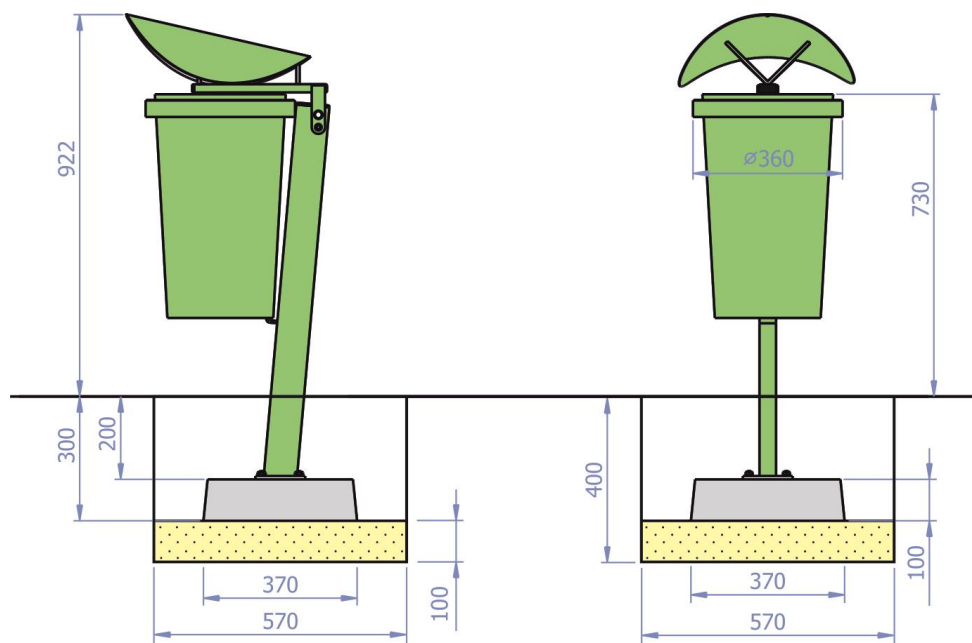
Rys.1 Schemat fundamentowania.
