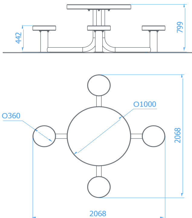
Wymiary urządzenia
