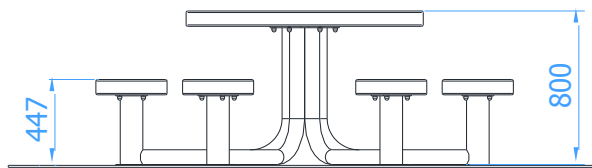
Wymiary urządzenia
