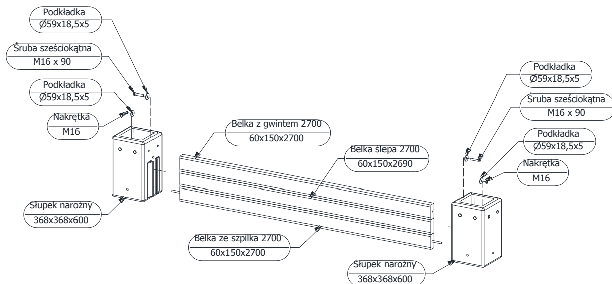
Rys. Schemat montażu belek długich (2690mm)
