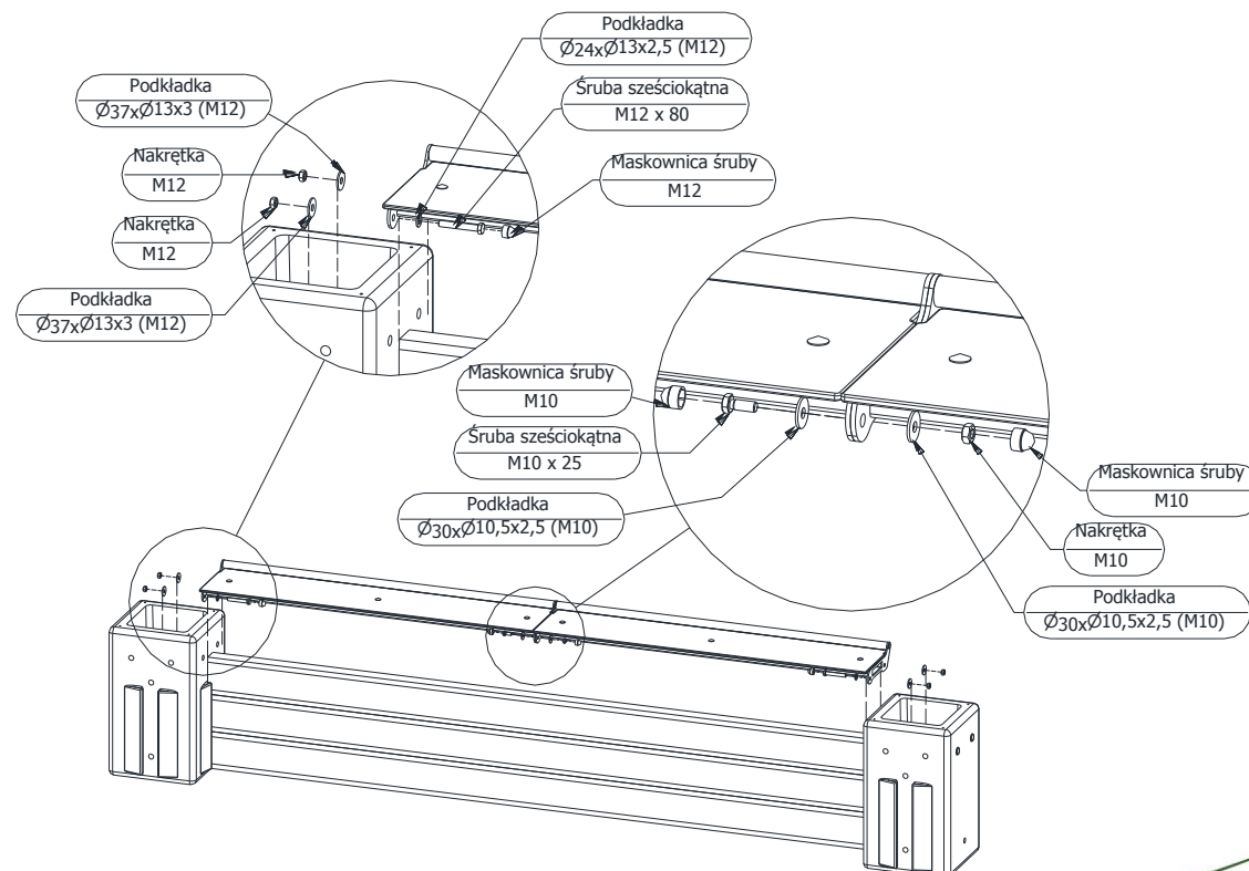
Rys. Schemat montażu siedziska długiego (2690mm)
