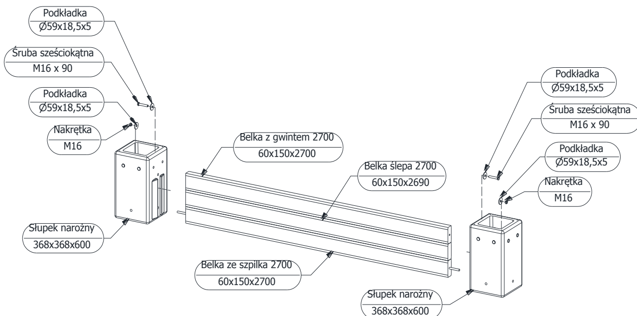
Rys. Schemat montażu belek długich (2690mm)
