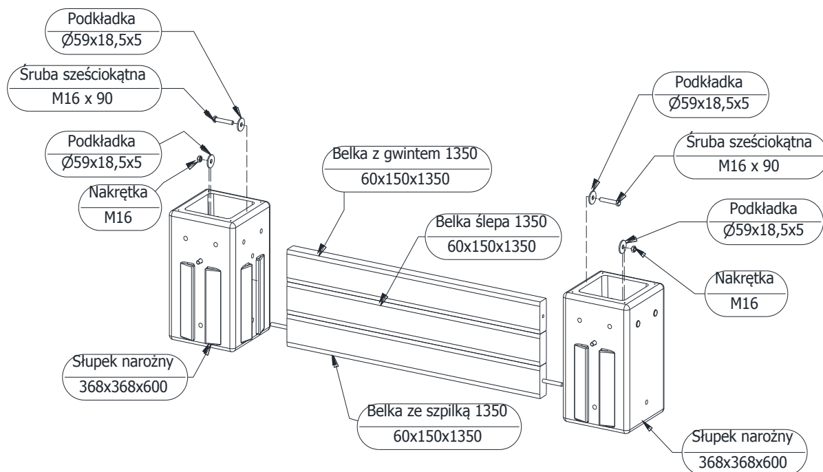
Rys. Schemat montażu belek krótkich (1350mm)
