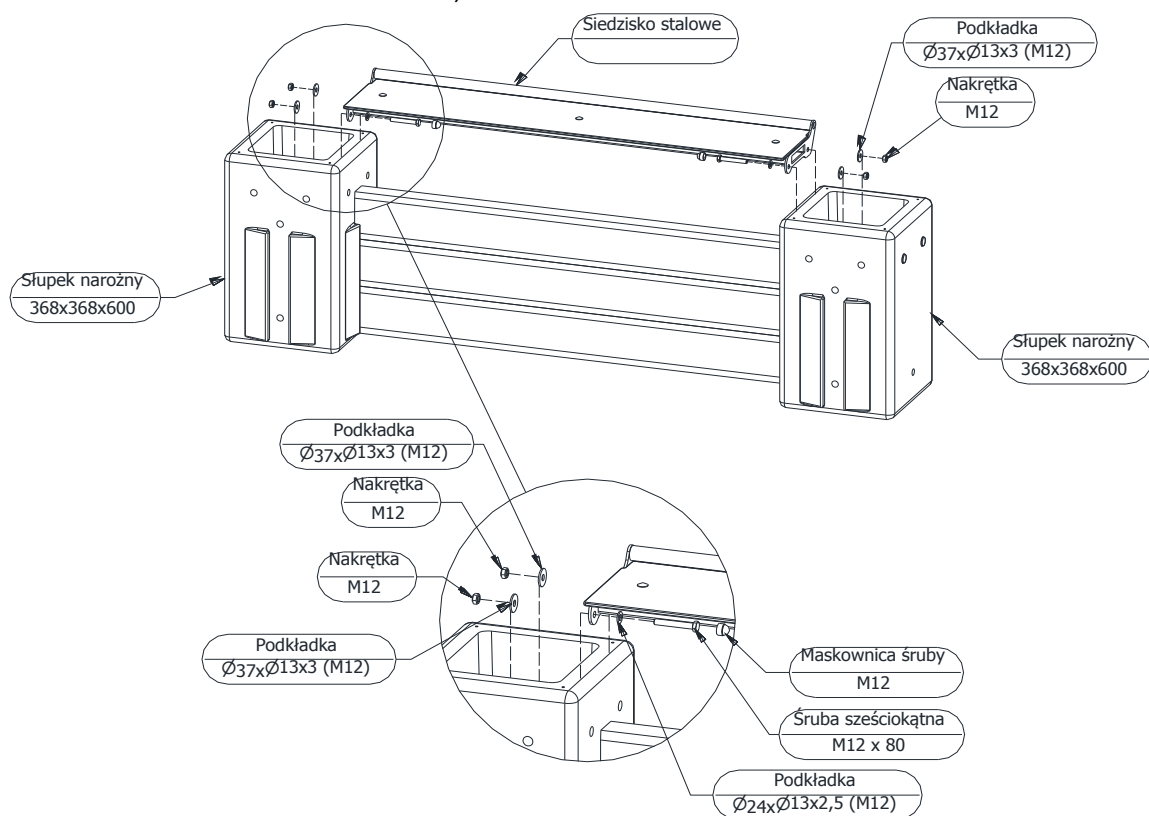
Rys. Schemat montażu siedziska krótkiego (1350mm)
